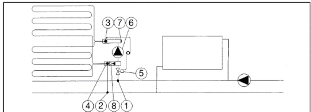
Principskema for tilslutning af Wirsbo kompaktshunt.
