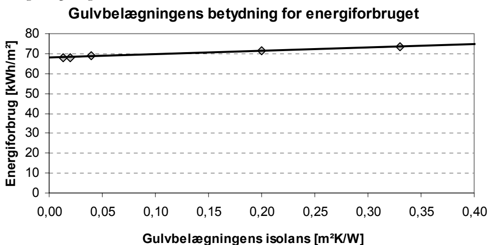
Figur 26 Simuleret varmeforbrug som funktion af gulvbelægningsens isolans
